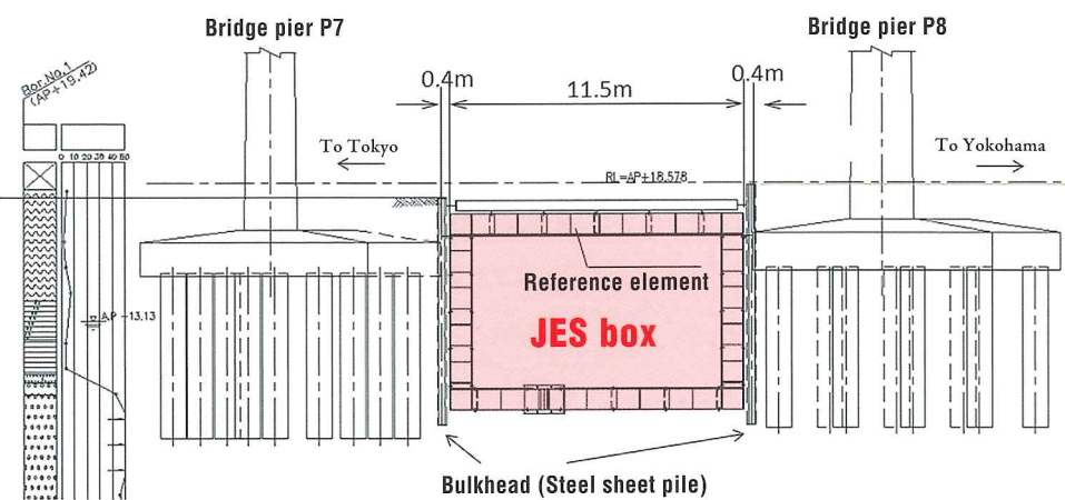
Fig. 1 Longitudinal profile
